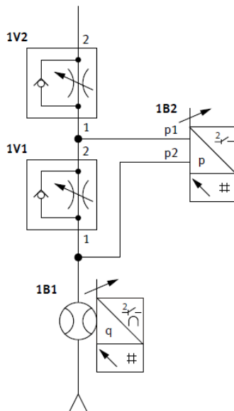
Esquema neumático
