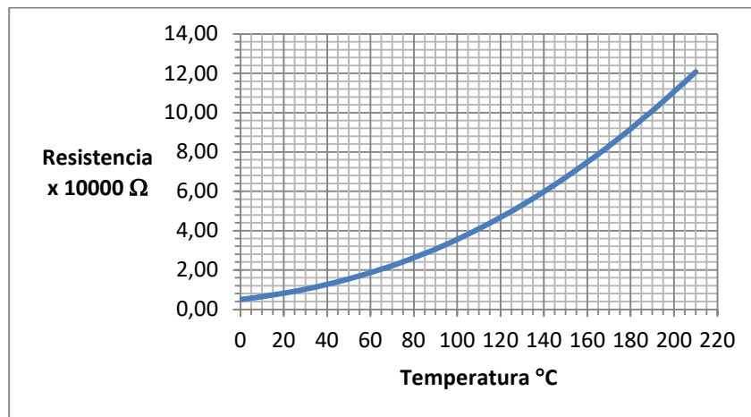
Característica Estática Gráfica de un PTC
