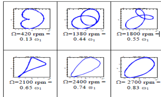
Orbitas descritas por el rotor desbalanceado y con eje agrietado para diferentes velocidades de rotación
